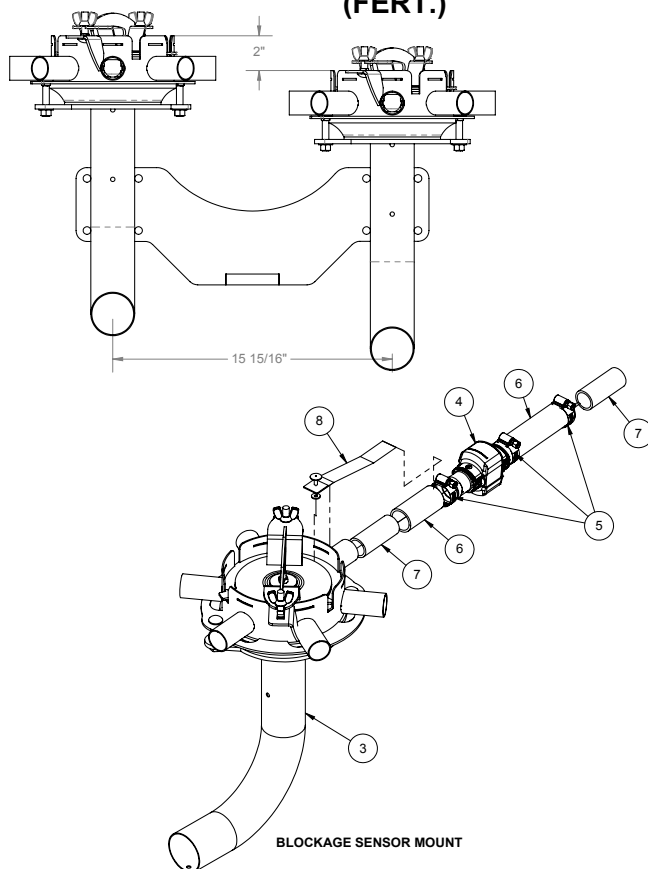
RIGHT MANIFOLD (FERT.)
