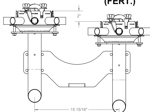
RIGHT MANIFOLD (FERT.)
